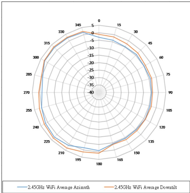
Azimet-Ebene (Draufsicht) - 2,45 GHz
