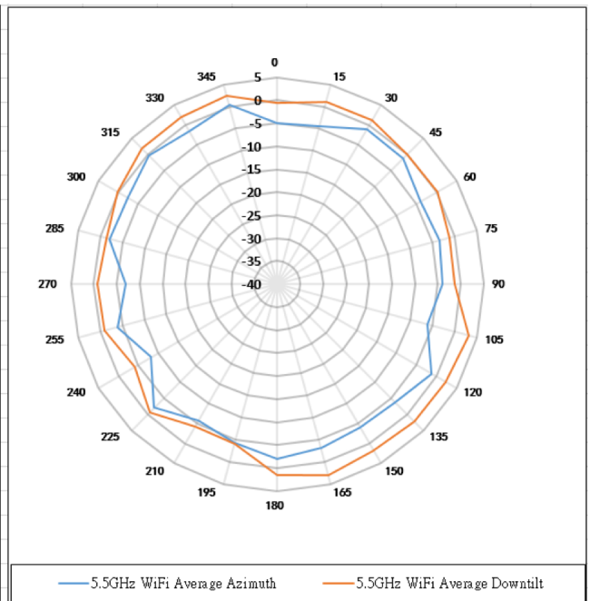
Azimet-Ebene (Draufsicht) - 5,5 GHz
